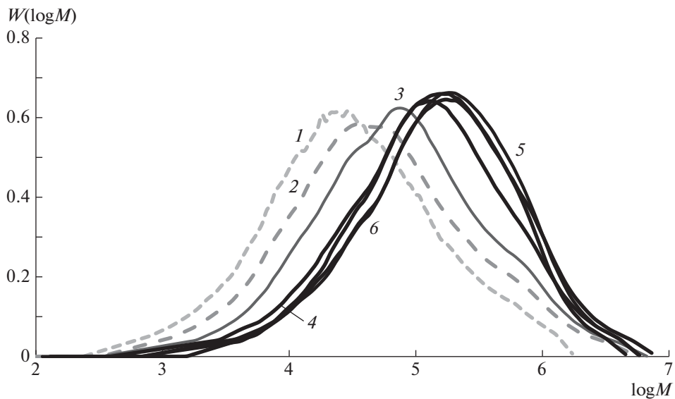
Рис. 4. Эволюция экспериментального ММР полибутадиена в ходе полимеризации. Время полимеризации 1 (1), 1.5 (2), 2.5 (3), 5 (4), 10 (5) и 90 мин (6).
