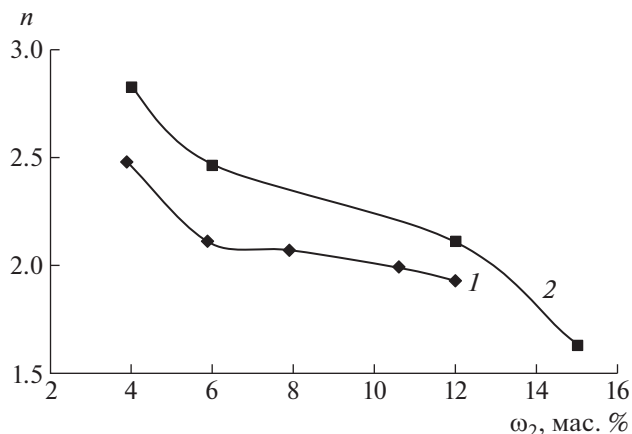
Рис. 5. Зависимость параметра n от концентрации ГПЦ и в смешанном растворителе вода/этанол с содержанием этанола 25 об. % (1) и в воде (2).
