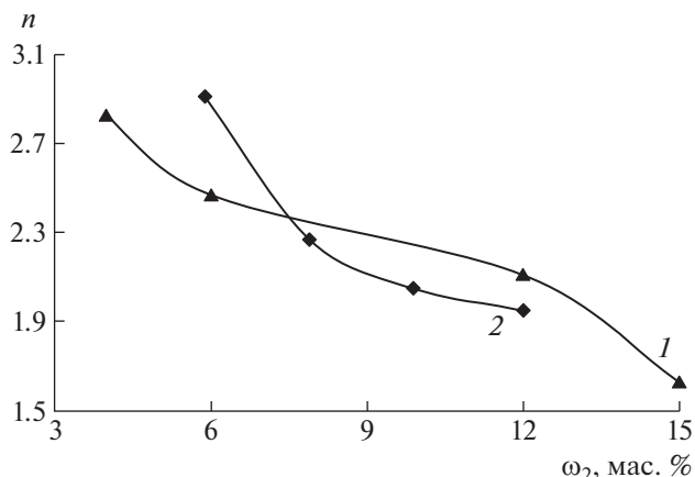
Рис. 6. Зависимость параметра n от концентрации ГПЦ в смешанных растворителях вода/этанол состава 50 : 50 (1) и 91 : 9 об. % (2).
